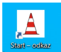
Obr. 2 - Spúšťanie aplikácie
